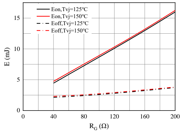
图 6. 开关损耗 逆变器
