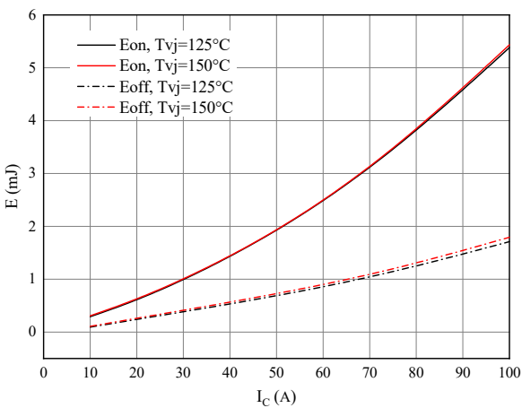
图 5. 开关损耗
