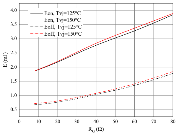
图 6. 开关损耗
